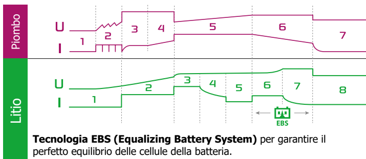
Curva di carica specifica in 7 tappe senza sorveglianza .
