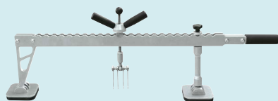
Dobbeltvirkende nivelleringsstang ref. 053564
